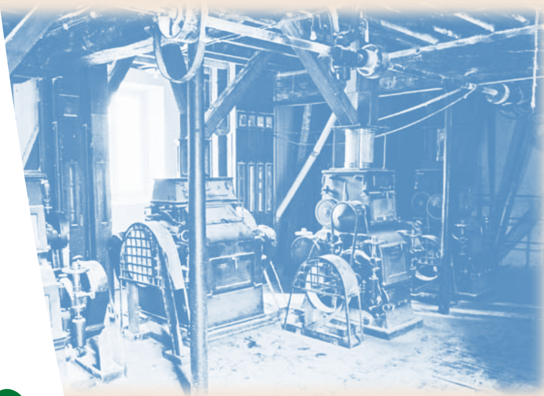
Broyeurs à cylindres © Photo M. Guevel
